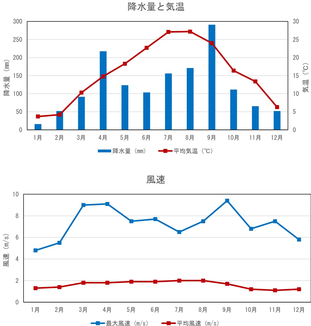
図1-5：国分寺市付近（府中市）の気象（資料：国土交通省気象庁/令和4年）
