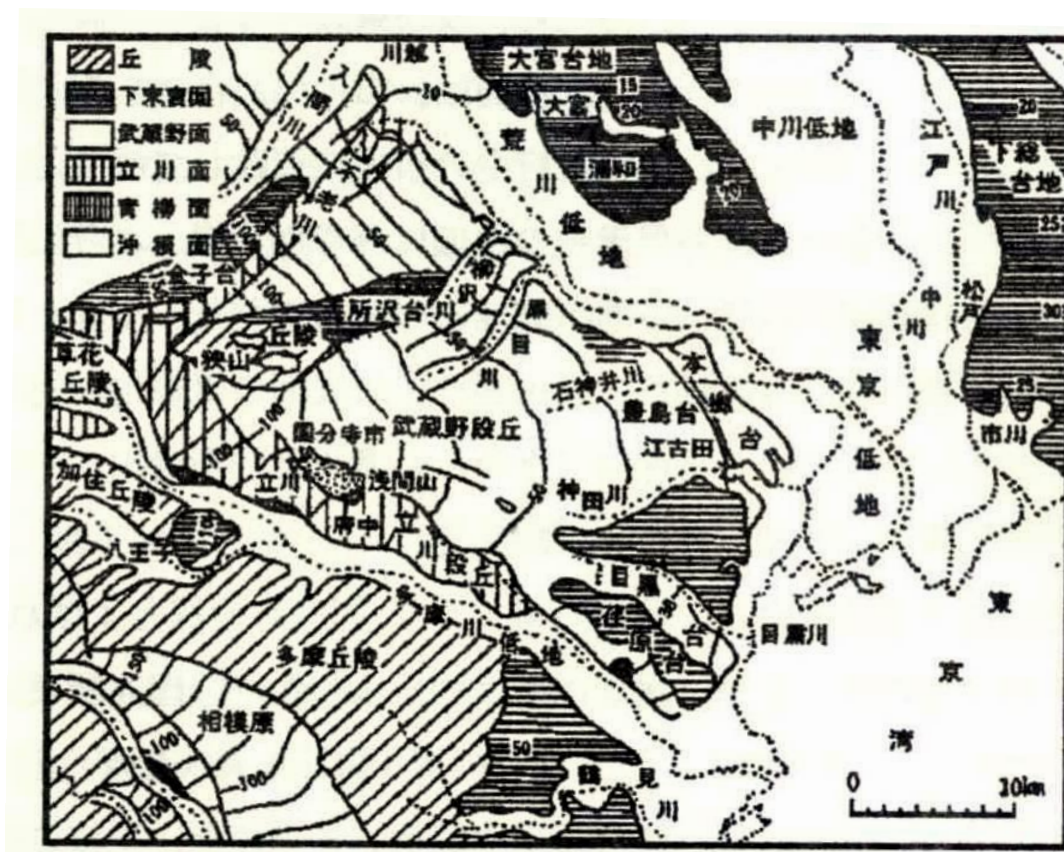
図1-2：武蔵野付近の地形区分と国分寺市の位置
