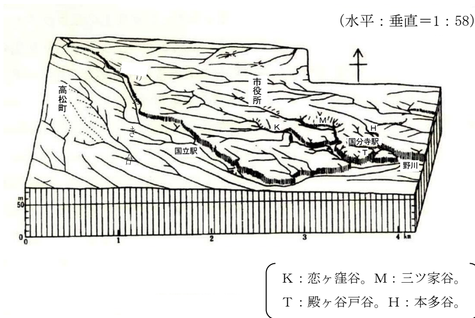
図1-3：国分寺市の地形ブロックダイヤグラム
